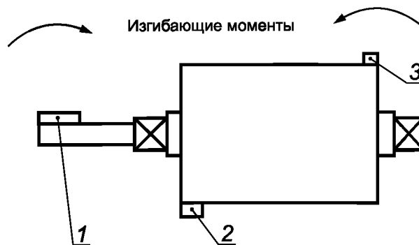
Рисунок D.1 — Внутренние моменты, создаваемые при компенсации дисбаланса, вызываемого полной шпонкой, двумя корректирующими массами на теле ротора
