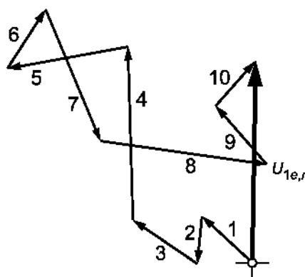
д) Результирующий эквивалентный модальный дисбаланс \vec{U}_{1e,r}
