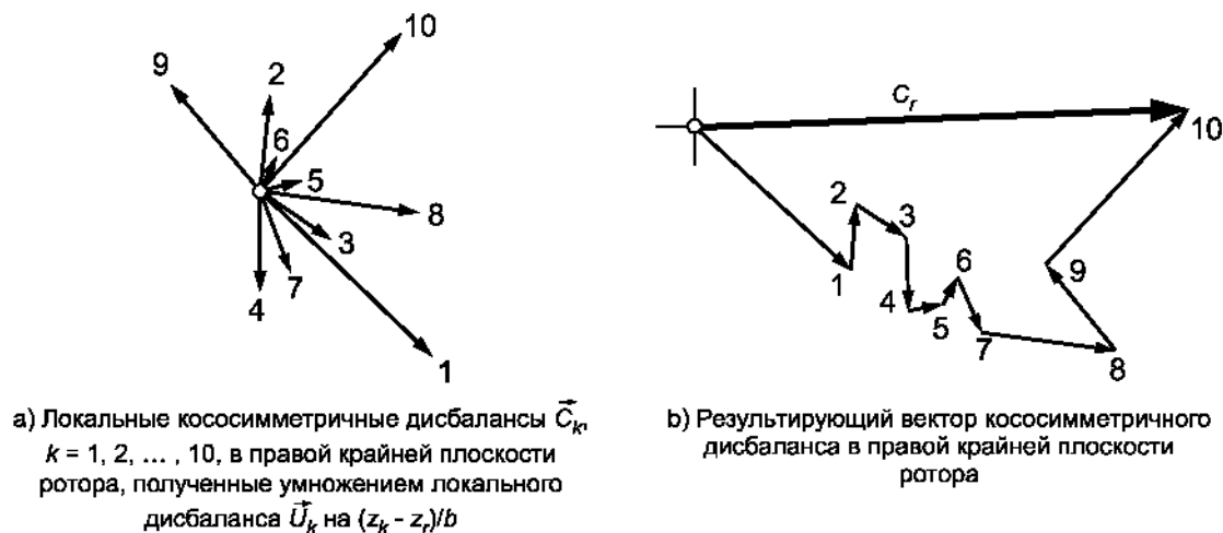
Рисунок А.6 — Графическое представление результирующего кососимметричного дисбаланса ротора
