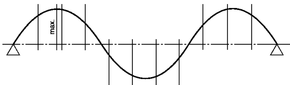
с) Третья мода изгибных колебаний \phi_3(z)
