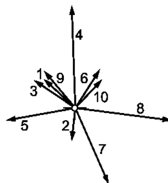
с) Локальные эквивалентные модальные дисбалансы \vec{U}_{1e,k}
